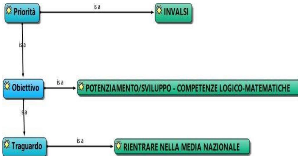
Figura 1: Priorità INVALSI
